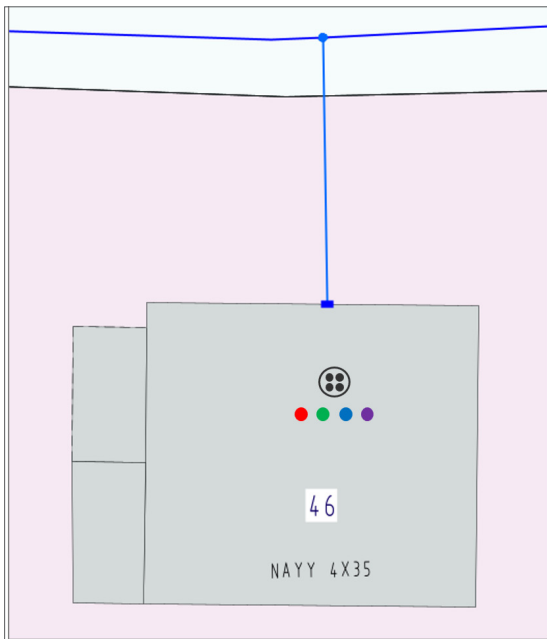
Mehrspartenhausanschluss mit Spartensymbolisierung und MSHE
