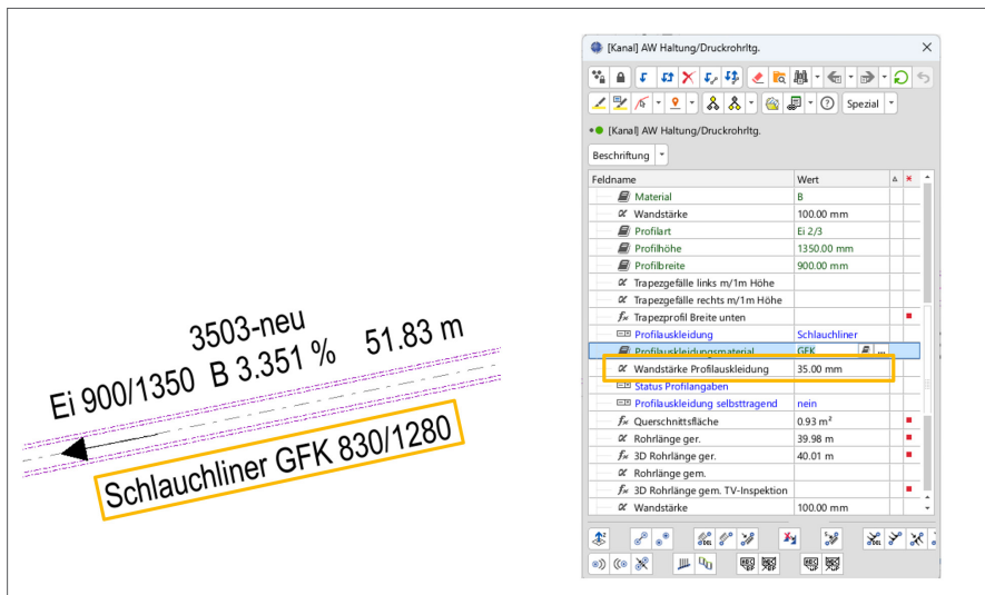
Haltung mit Beschriftung des Sanierungsprofils
