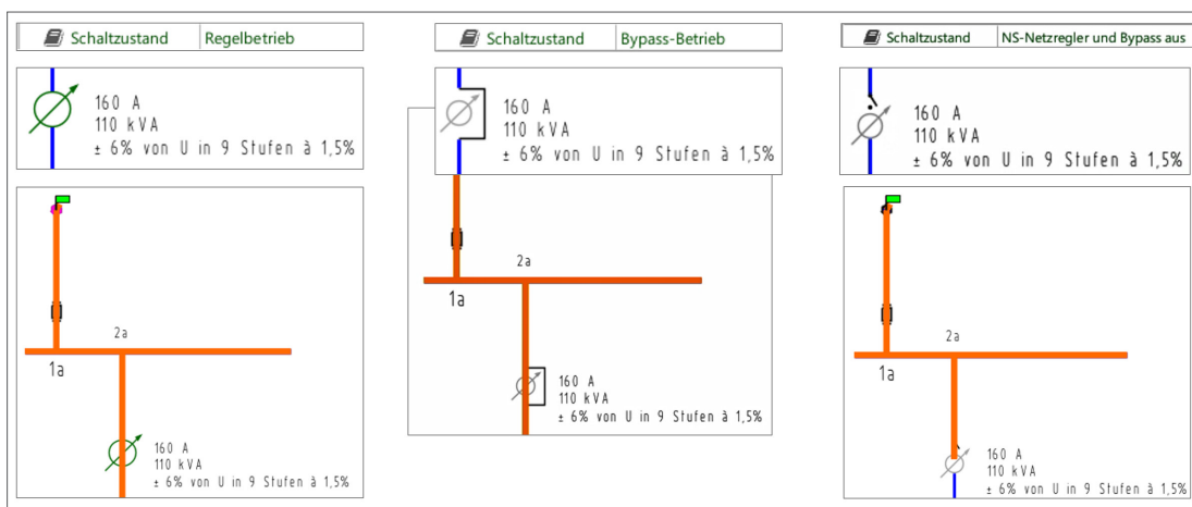
Schaltzustände des NS-Netzreglers
